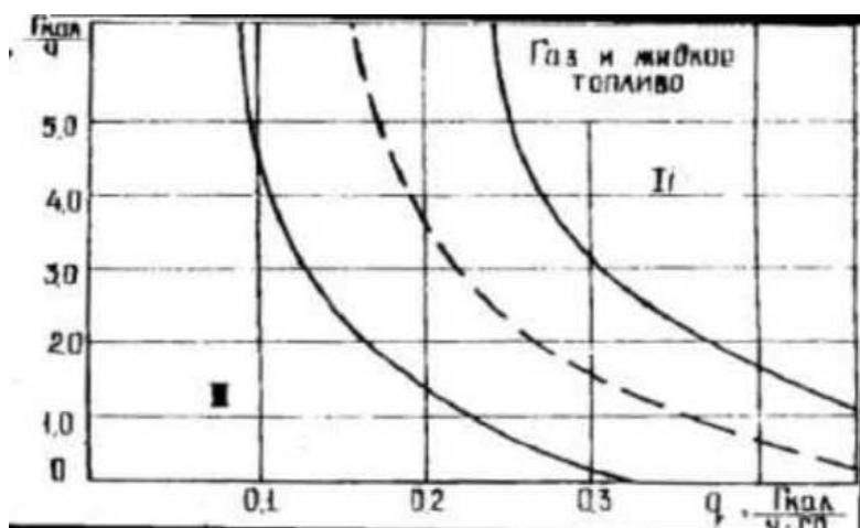
Рис. 3. Ориентировочные значения области устойчивой экономичности централизованного (II) и децентрализованного (I) теплоснабжения.
